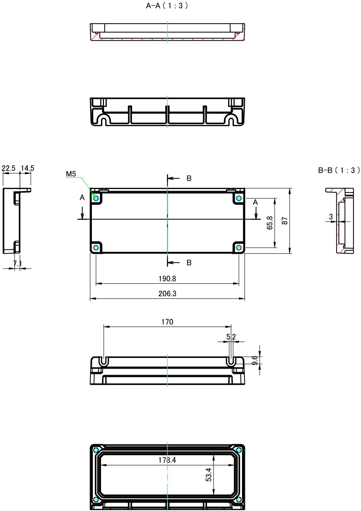
フランジ付側板1 Fianged end panel 1
