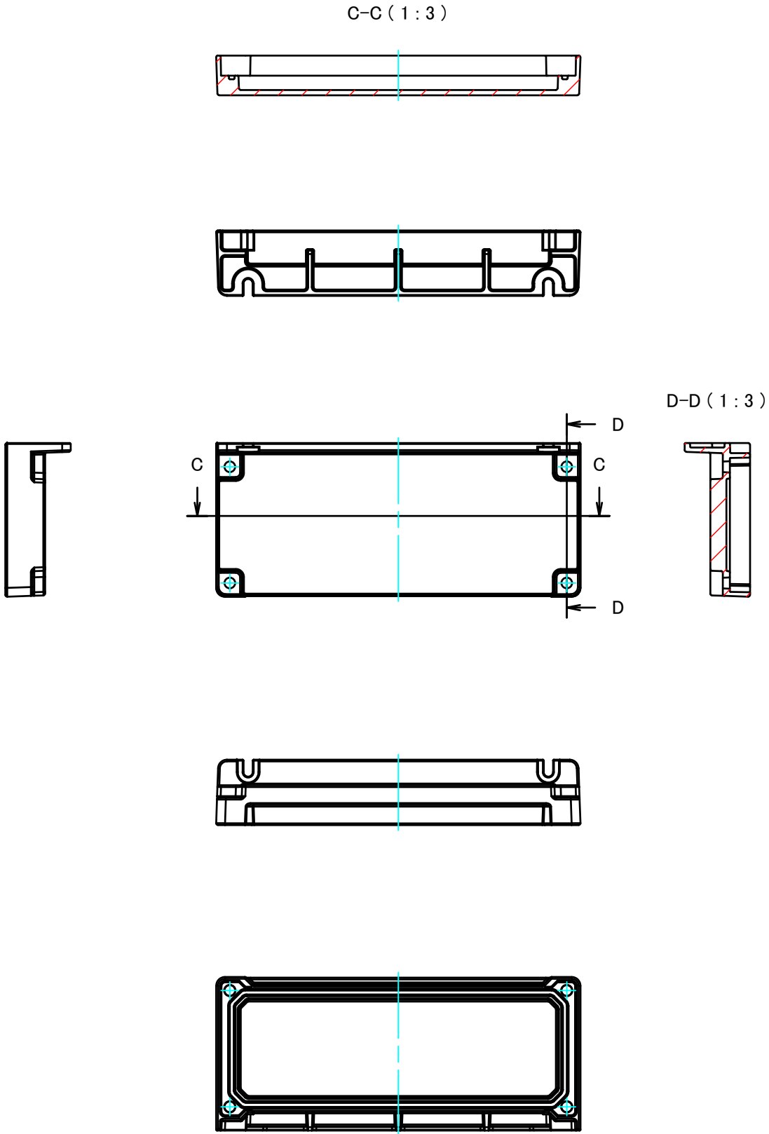
フランジ付側板2 Fianged end panel 2
